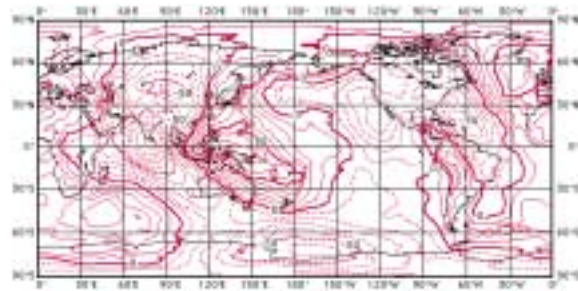
図 20: 全世界のジオイド高の分布 (出典: 理科年表)
