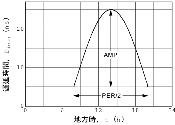
図 9: 電離層遅延モデル
