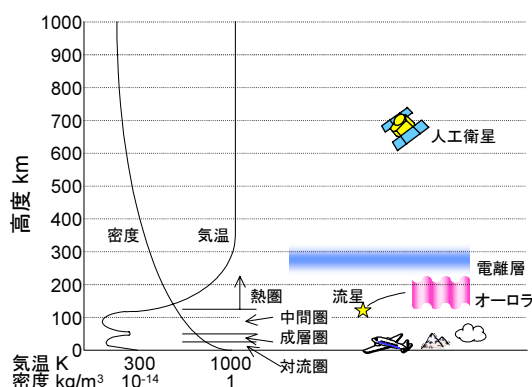
図 12: 高層大気圏の構造
