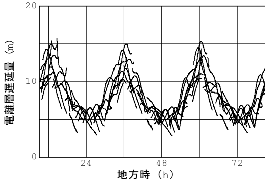
図 13: 電離層遅延の実測例 (2002 年 9 月 22～24 日, 調布市)
